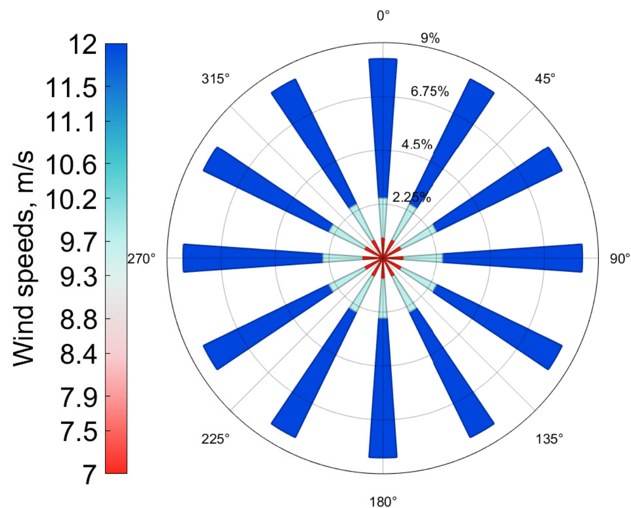
Wind Scenario 4
